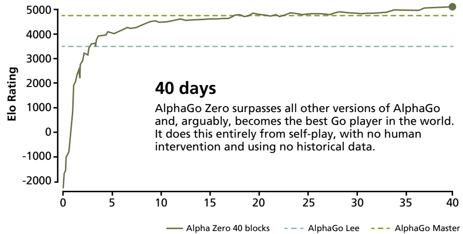
Abbildung 7 Lernfortschritt von AlphaGo Zero mit bestär- kendem Lernen [15]
